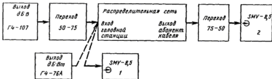
Рис. 7.11. Структурная схема измерения отношения сигнала к шуму
