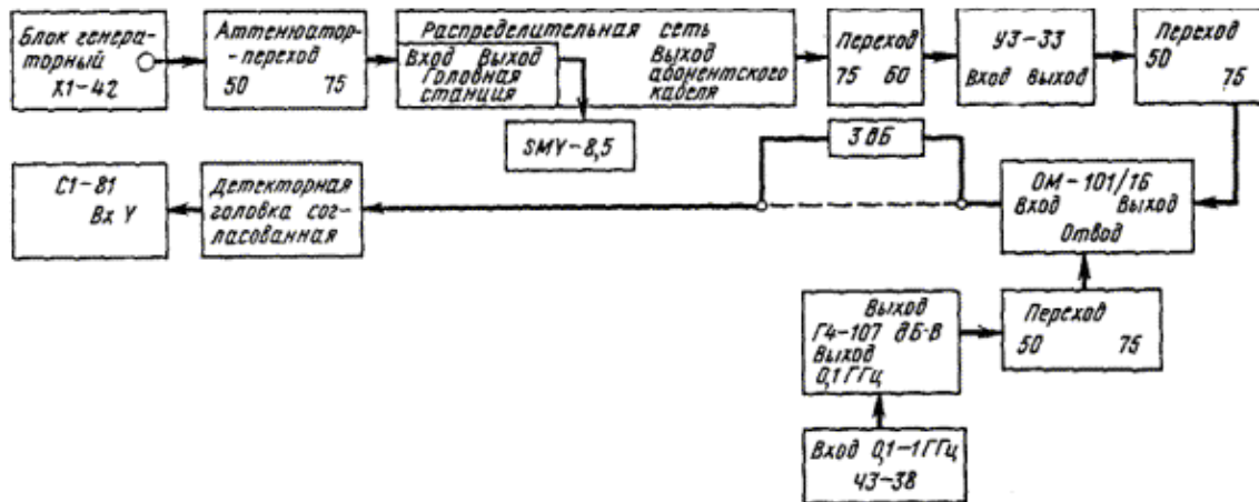
Рис. 7.1. Структурная схема измерения неравномерности АЧХ
