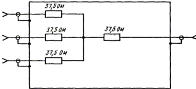
Рис. 7.6. Принципиальная схема согласующего устройства
