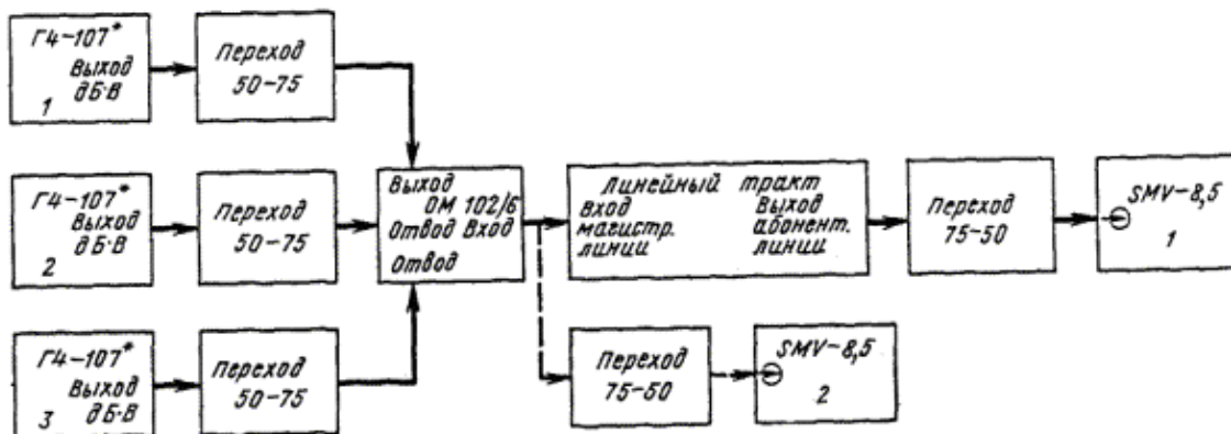
Рис. 7.7. Структурная схема измерения отношения сигнала к помехе комбинационной частоты третьего порядка IMAIII(в)
