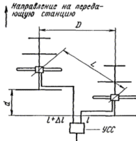
Рис. П.1.2. Сдвоенная антенна со сдвигом
