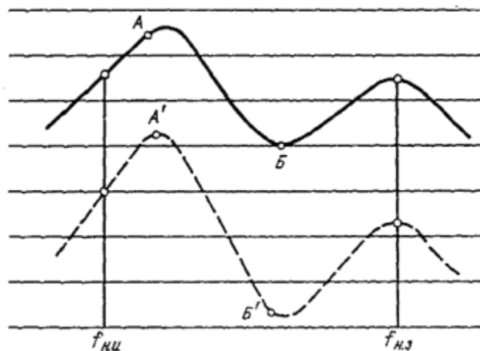
Рис. 7.2. Пример изображения АЧХ на экране осциллографа
