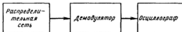
Рис. П.3.1. Схема измерения импульсной характеристики
