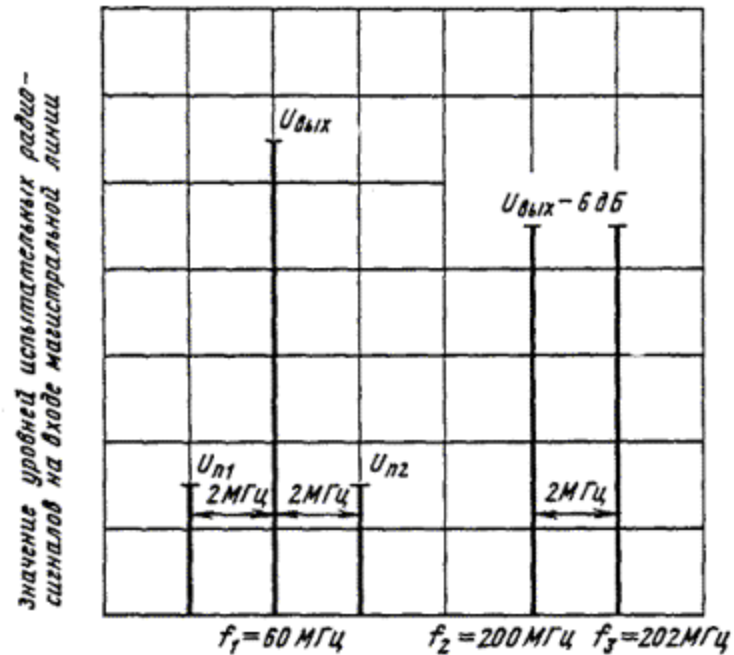
Рис. 7.8. Соотношение уровней сигналов на входе линейного тракта при измерении ИМАШ(в)
