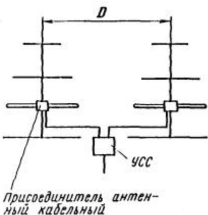
Рис. П.1.1. Сдвоенная антенна
