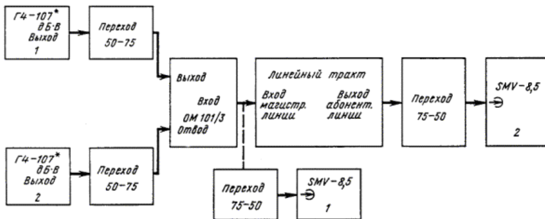
Рис. 7.10. Структурная схема измерения отношения сигнала к помехе комбинационной частоты второго порядка I_{MAII(B)}
