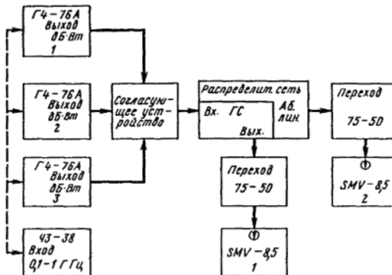
Рис. 7.5. Структурная схема измерения сигнала к помехе комбинационной частоты третьего порядка ИАШ(к) в дециметровом диапазоне
