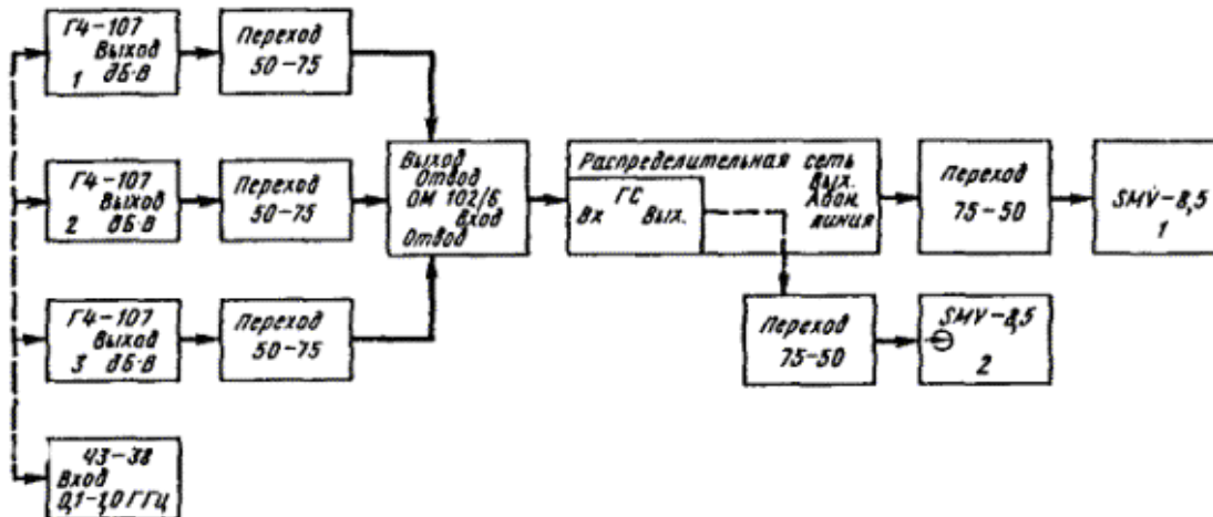
Рис. 7.3. Структурная схема измерения отношения сигнала к помехе комбинационной частоты третьего порядка IMAIII(к) в метровом диапазоне волн
