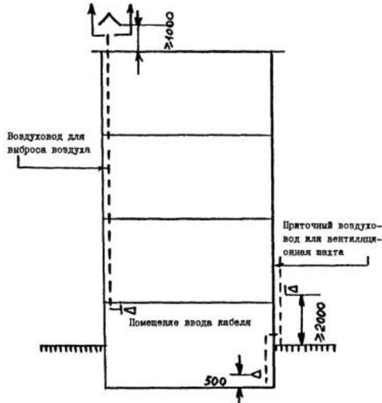
Рис. 1. Принципиальная схема вентиляции помещения ввода кабеля.
